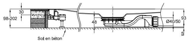
Dessin avec vidage B597- BetteSolid 30 - 0,6 l/s, hauteur de garde d'eau: 30 mm
