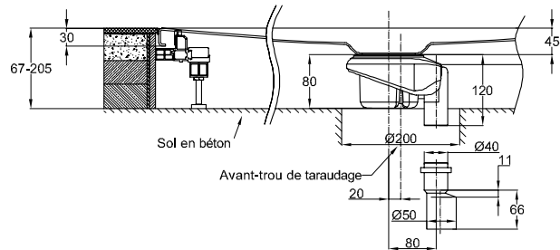
Dessin avec vidage B573- BetteDown - 0,6 l/s, hauteur de garde d'eau selon les normes: 50 mm
